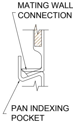
DETAIL C - SCALE: N.T.S. PAN JOINT DETAIL
